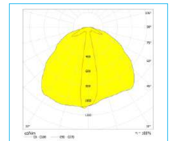
120x25°
