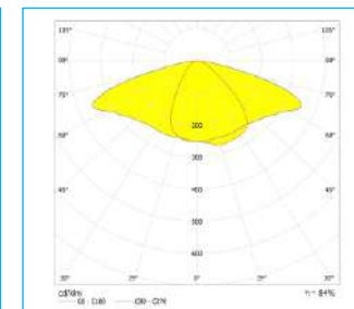
80x150°
